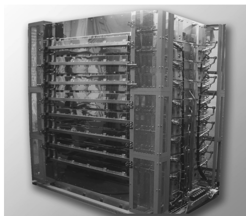
自動車用多段式鋼板加熱装置 (高張力鋼板を約1000℃まで短時間で加熱します)
