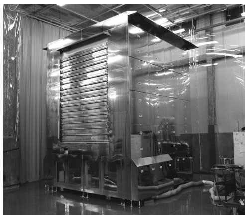
FPD用多段式熱処理装置 (LCDガラス基板の焼成・アニール・乾燥等 クリーンな環境での熱処理装置です)
