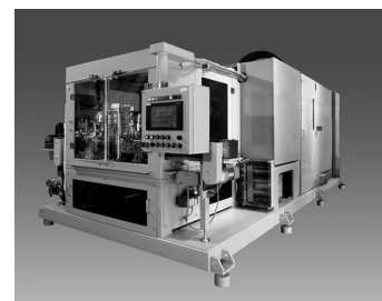
インデックス方式の高速加工 高周波焼入焼戻設備
