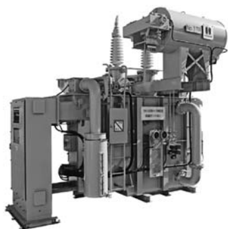
図1 環境調和型変圧器（ナタネ油入負荷時タップ切換変圧器）
