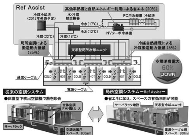
冷媒自然循環式局所冷却システム
