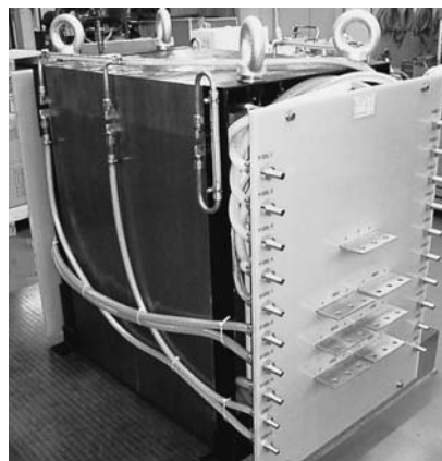
商用周波変圧器 (60Hz3750kVA)
